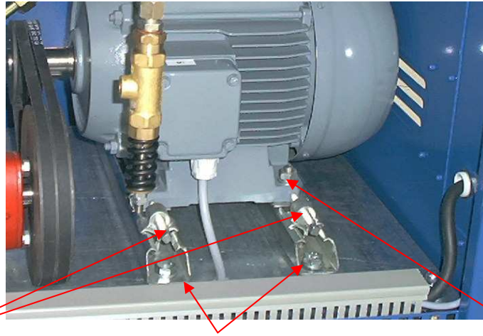
Spannschienen
