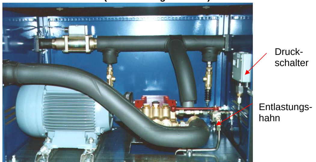
Vorderseite (Auslieferungszustand)
