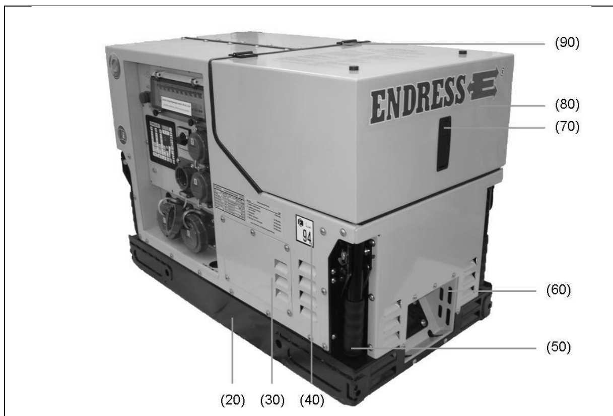
Abb. 9-1: Schalldämmhaube
