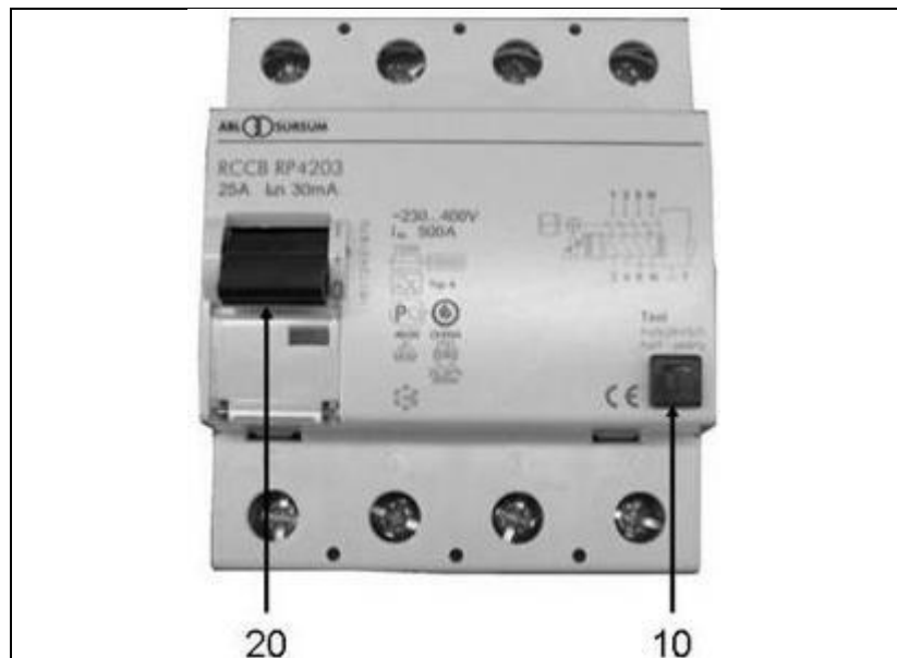
Abb. 5-1: FI-Schutzschalter
