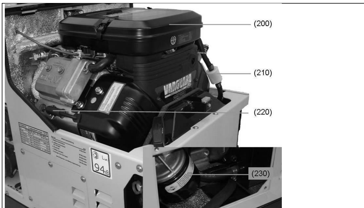
Abb. 9-3: Ersatzteile Motor
