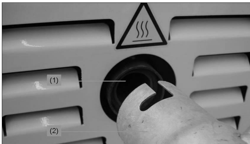
Abb. 5-13 Abgasschlauch anschließen
