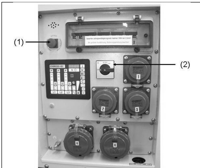
Abb. 4-2: Bedienpaneel Standardausführung
